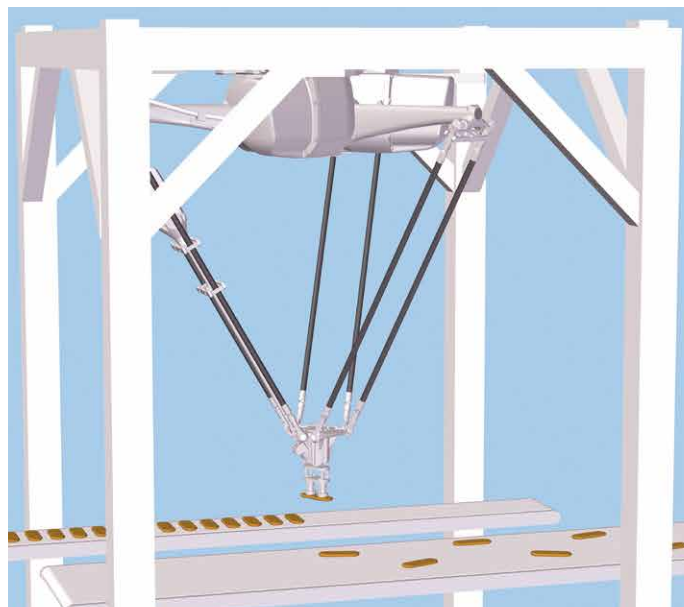
DR-3 i B/8Lによる食品の高速整列
