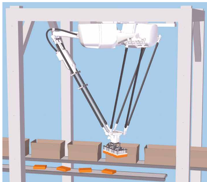
DR-3 i B/8Lによる高速食品箱詰め
