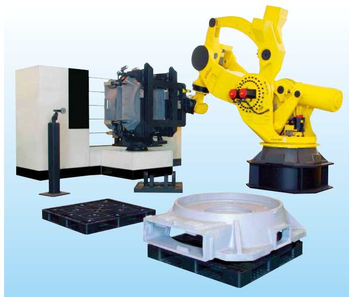
M-2000iA/1200による大型鋳物の加工用治具へのセット
